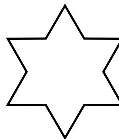
sześciokąt gwiaździsty foremny
